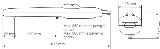
Tabulka 2: Bez vnitřního pevného dorazu, s max. 350mm pojezdem
